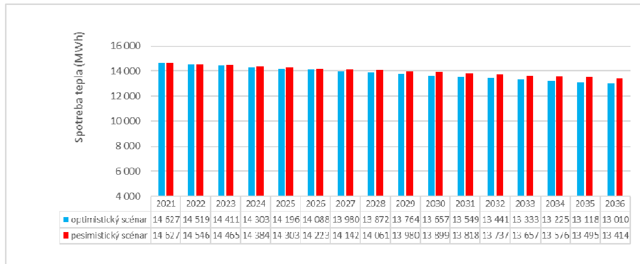
Graf 17: Scenáre predpokladaného vývoja spotreby tepla na Sídlišku pod Sokolejom v horizonte nasledujúcich 15 rokov
