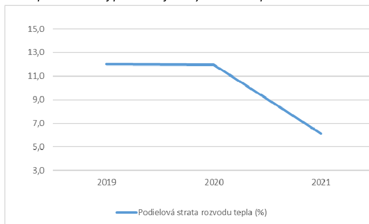
Graf 10: Priebeh percentuálnej podielovej straty rozvodu tepla za obdobie rokov 2019-2021
