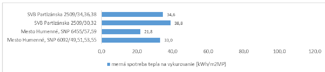
Graf 16: Merné spotreby tepla na vykurovanie v roku 2021 správcov SVB a Mesto Humenné
