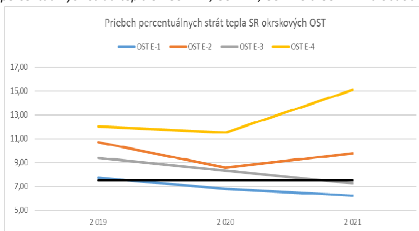
Graf 12: Priebeh percentuálnych strát tepla SR OST E-1, OST E-2, OST E-3 a OST E-4 za obdobie rokov 2019-2021
