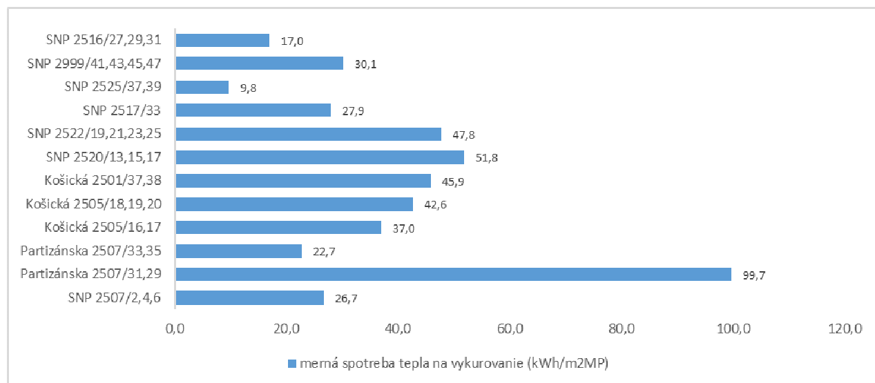
Graf 15: Merné spotreby tepla na vykurovanie v roku 2021 správcu ENERGOBYT s.r.o. Humenné
