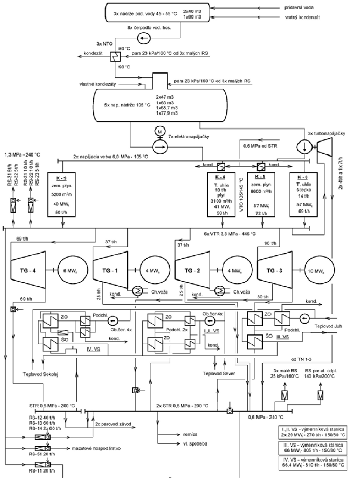
Obrázok 3: Situačná schéma zapojenia technologických zariadení na výrobu tepla a elektrickej energie v teplárni CHEMES, a.s. Humenné
