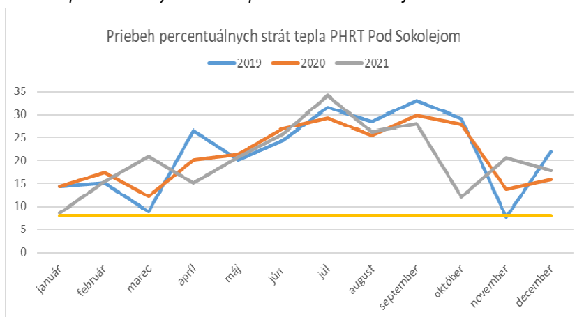
Graf 11: Priebeh percentuálnych strát tepla PHRT Pod Sokolejom za obdobie rokov 2019-2021
