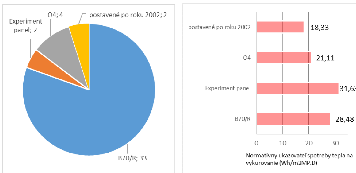
Graf 5: Štruktúra bytových objektov podľa stavebných sústav a normatívny ukazovateľ spotreby tepla na vykurovanie bytových objektoch uvedených stavebných sústav
