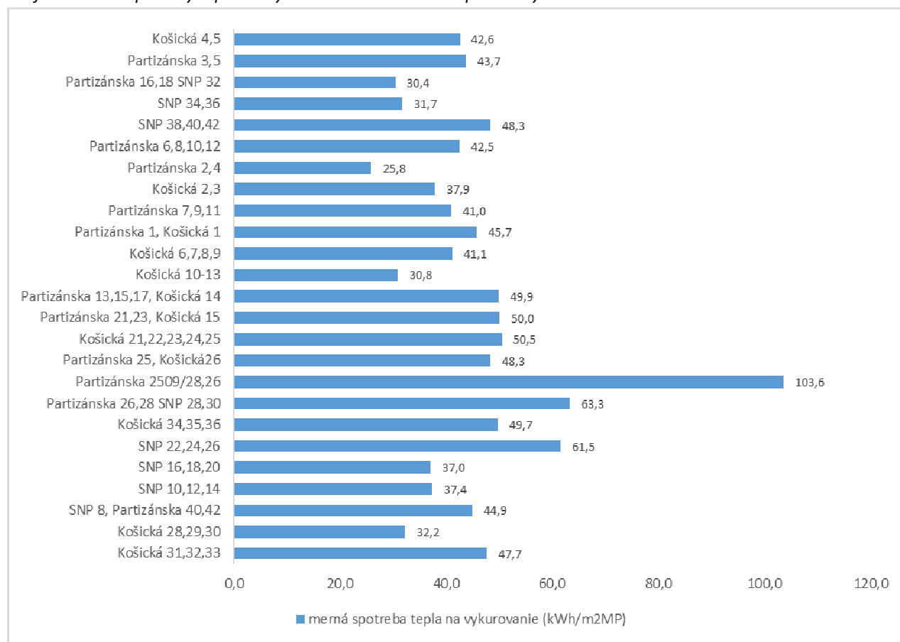
Graf 14: Merné spotreby tepla na vykurovanie v roku 2021 správcu Bytové družstvo Humenné
